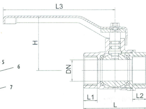
KULOVÝ KOHOUT PLNOPRŮTOKOVÝ
