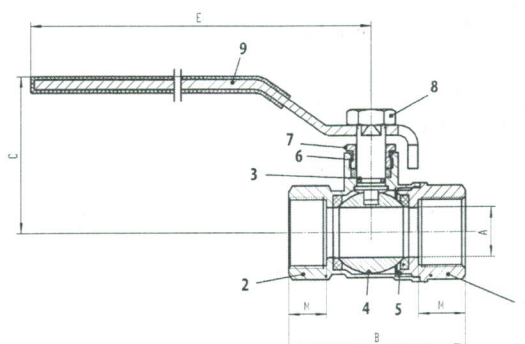
KULOVÝ KOHOUT PLNOPRŮTOKOVÝ TĚSNĚNÝ TEFLONOVOU UCPÁVKOU
