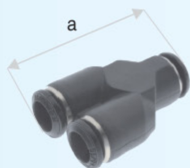
55310 - SPOJKA HADIC Y
