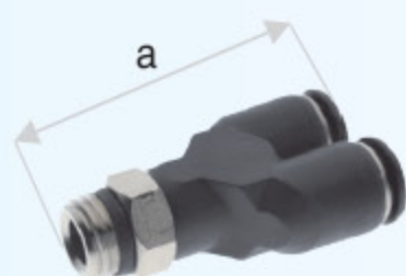
55320 - SPOJKA HADIC Y
