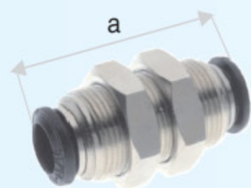
50050N - SPOJKA PŘES PŘEPÁŽKU
